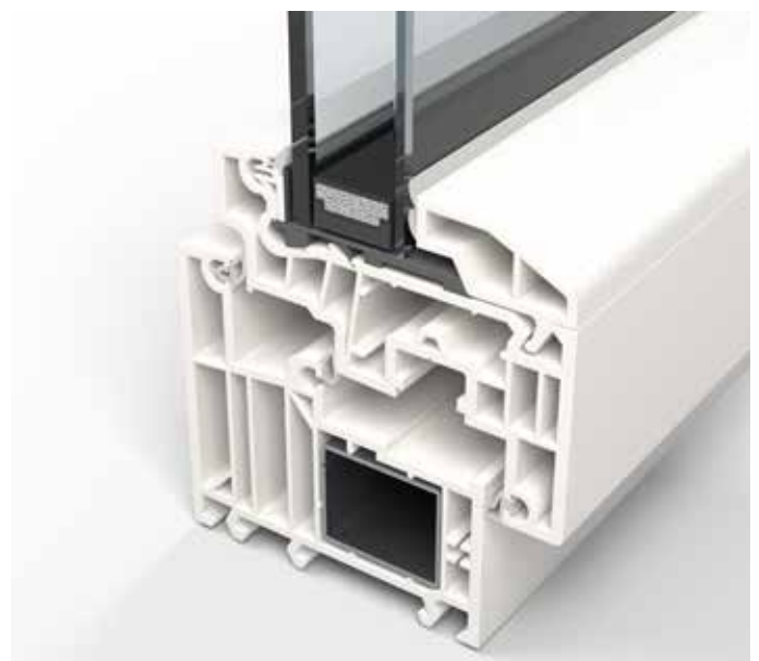
doorsnede van een raam met dubbel isolatieglas, opbouw 4v-18-6F
