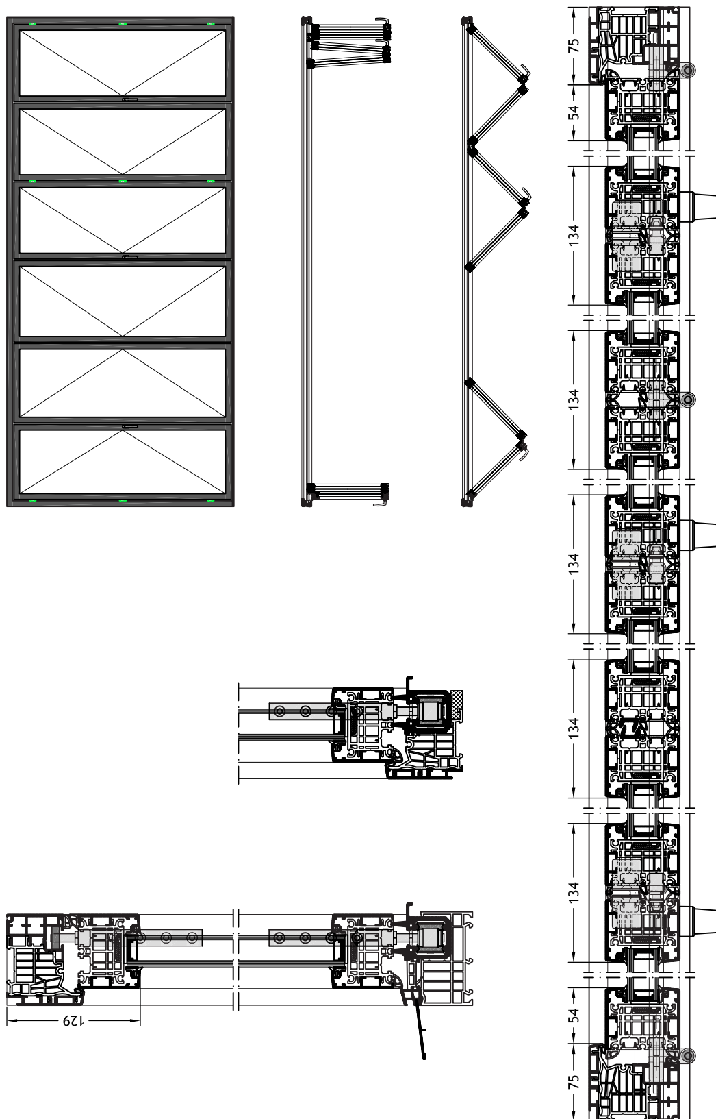
Frame G12 met vleugel Slim-line C40
